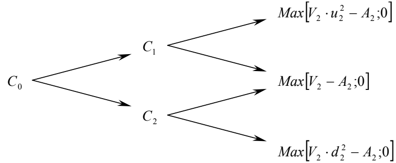
Figura 2: Valor conjunto de dos opciones de ampliación según método binomial multiplicativo.
